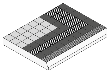
Mittelteil mit Leitstreifen und Auffindestreifen DIN 32984 und H-BVA (Länge 300 cm x Breite 223 cm)
