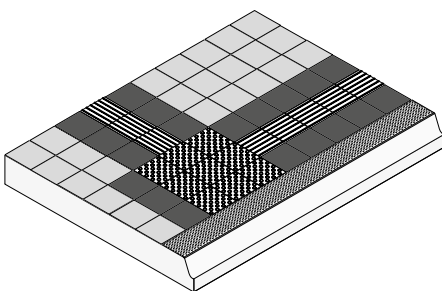
Mittelteil mit Einstiegsfeld und Leitstreifen nach Leitfaden Straßen.NRW (Länge 300 cm x Breite 223 cm)
