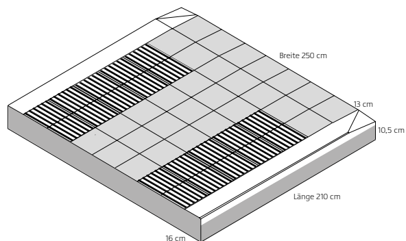
Mittelteil für getrennte Querung 6-3-0 Sehbehinderte mit 6 cm Tastkante
