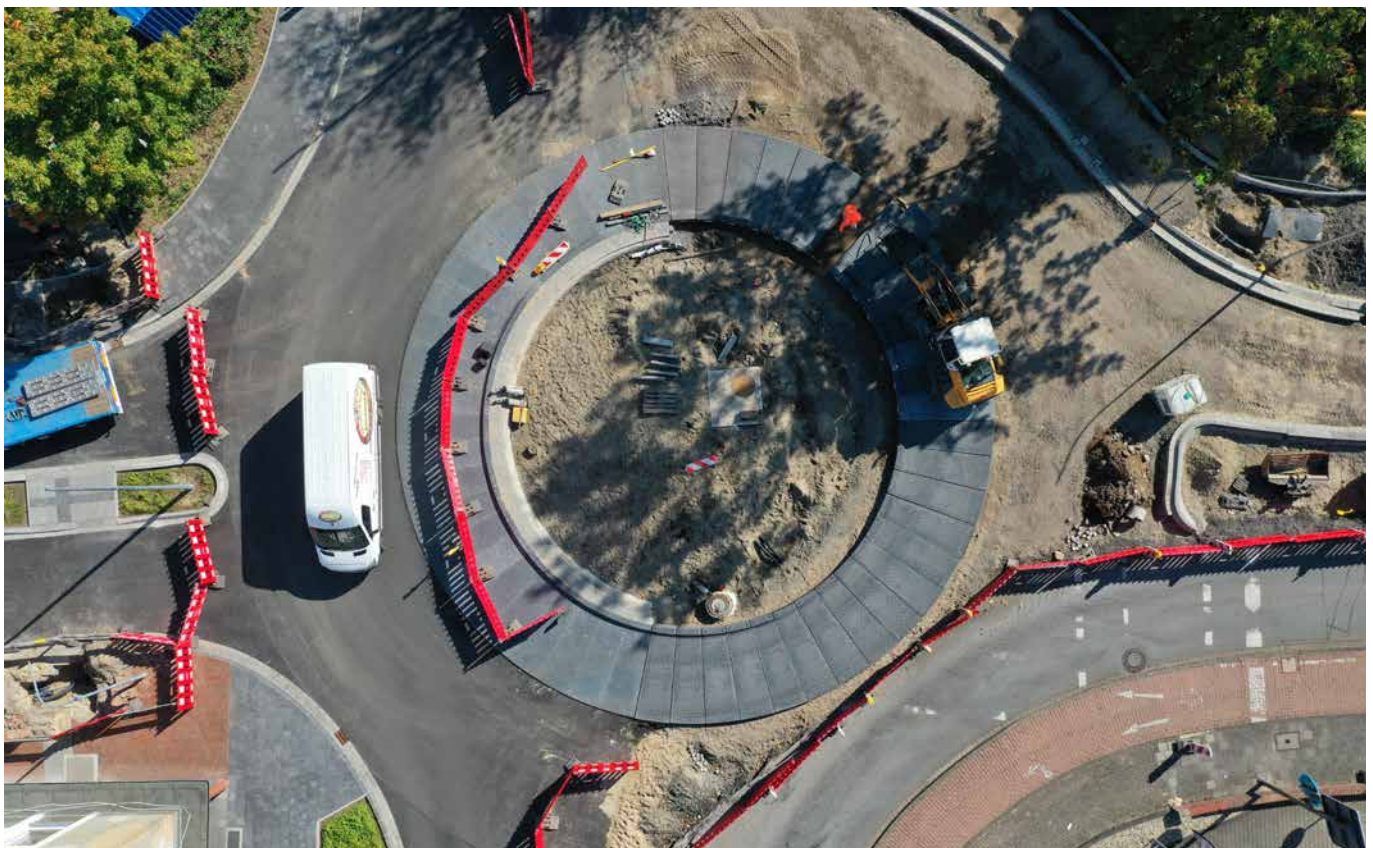
Versetzen eines MONODUR®-Kreisverkehrs mit halbseitiger Verkehrsführung
