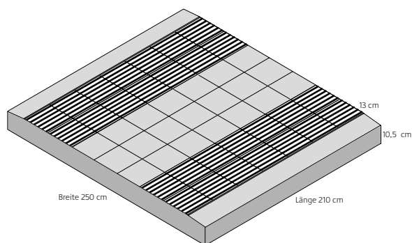
Mittelteil für getrennte Querung 3 cm Nullabsenkung für Gehbehinderte
