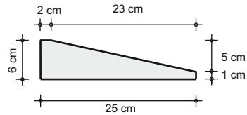
Querschnitt Rampenstein
