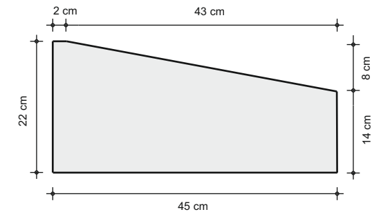
Querschnitt Schrägbord
