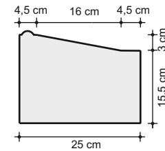
Querschnitt Easycross
