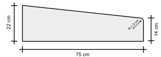
Querschnitt Schrägbord
