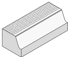
Busbord 43,5/31 cm Anlaufhöhe 16 cm (Baulänge 1 m)
