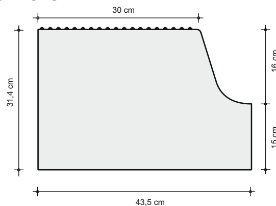
Rundkopfstein für Buskap senkrechter Anschluss rechts (Baulänge 1 m)
