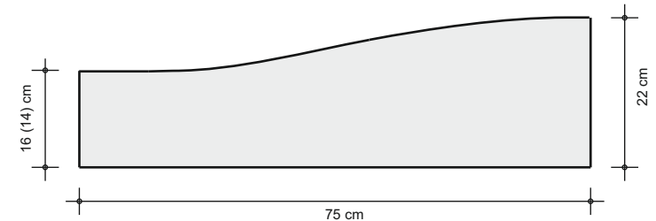
Querschnitt Rampenstein
