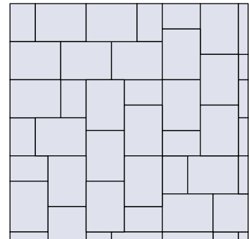
Blockverband 20 x 15 cm + 15 x 10 cm
