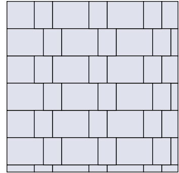
Reihenverband mit 2 Formaten 20 x 15 cm + 15 x 10 cm
